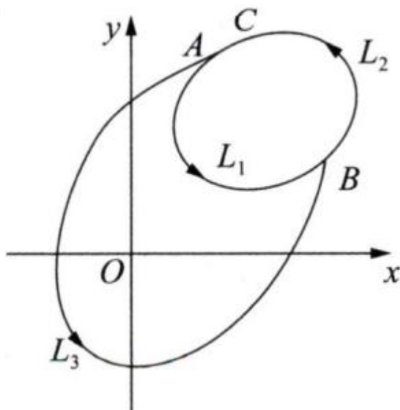
三(19)题图 (II) 因为对任意右半平面的闭曲线 C 都有
